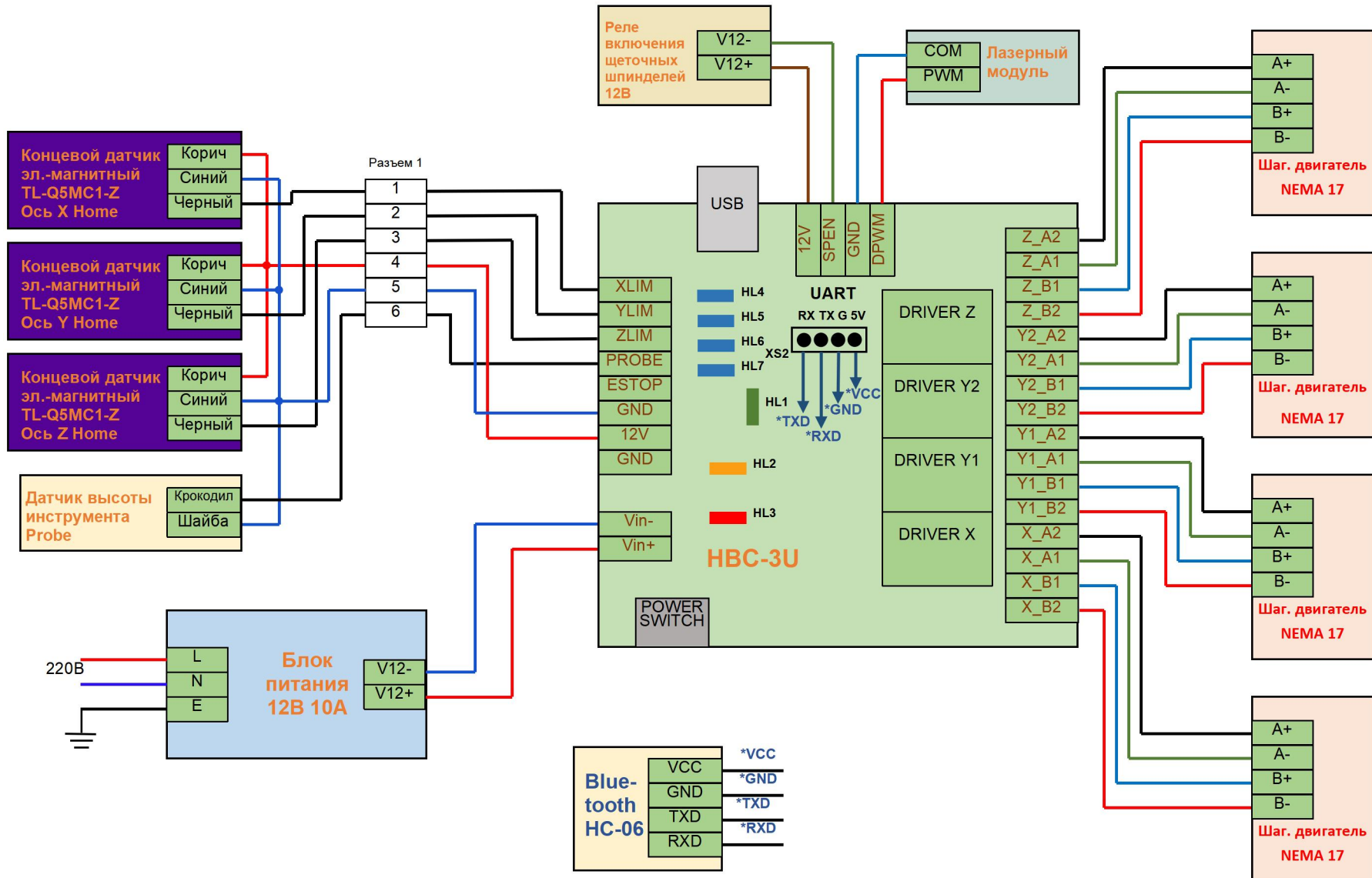
Схема подключения ЧПУ-контроллера HBC-3U к станку
